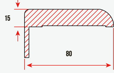
Örnek Pervaz Modeli/Frame Model
