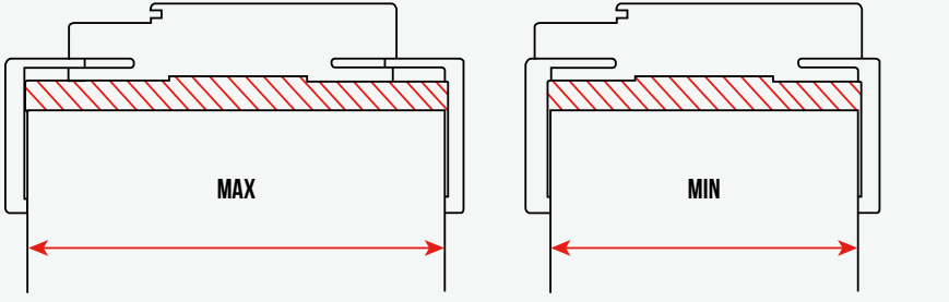
Pervaz Çalışma Payları/Frame Working Margins (0-60 mm)
