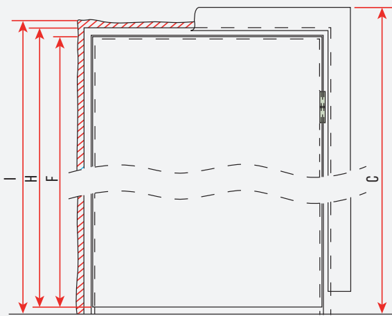
RESİM/PICTURE 2: KAPI YÜKSEKLİKLERİ/HEIGHT OF DOOR
